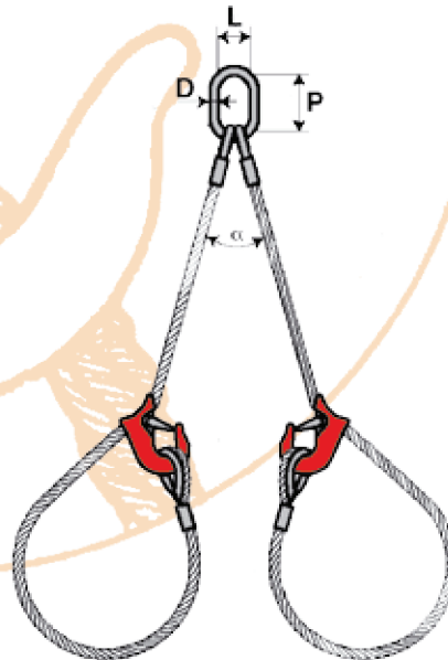
T2GS Brache scorsoi a due tratti Choker sling two legs
