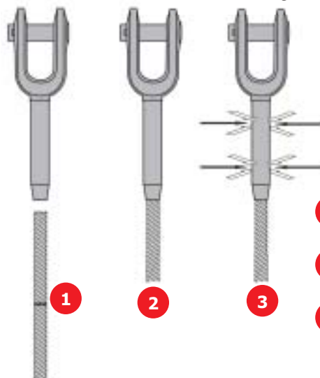
Capocorda terminale a pressare / Swage Socket
