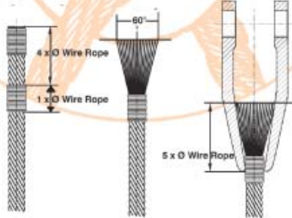
Capocorda terminale a pressare / Swage Socket
